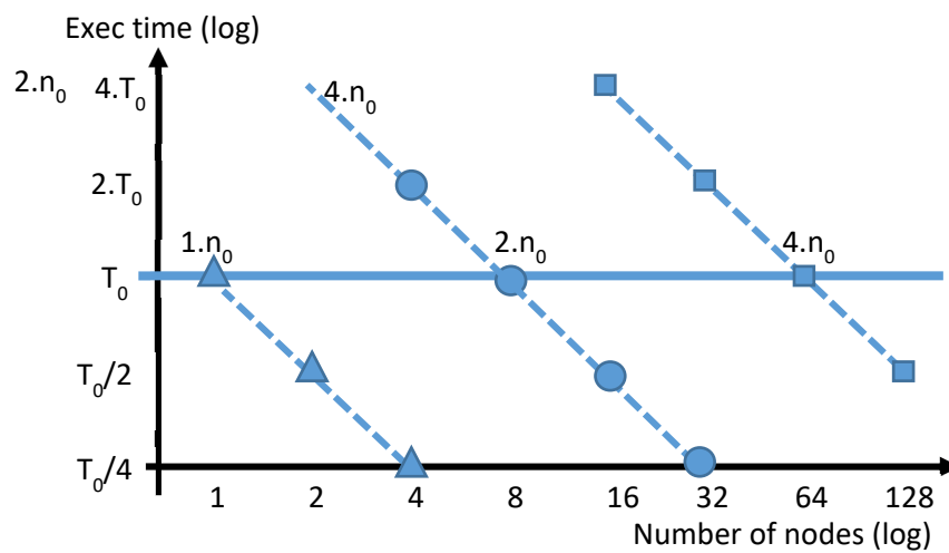
Figure 2 : abaque de temps d'exécution du code client
