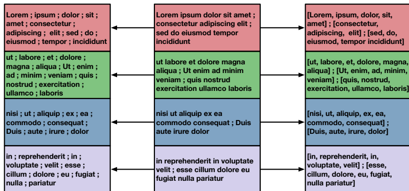
flatMap(lambda x: x.split())
